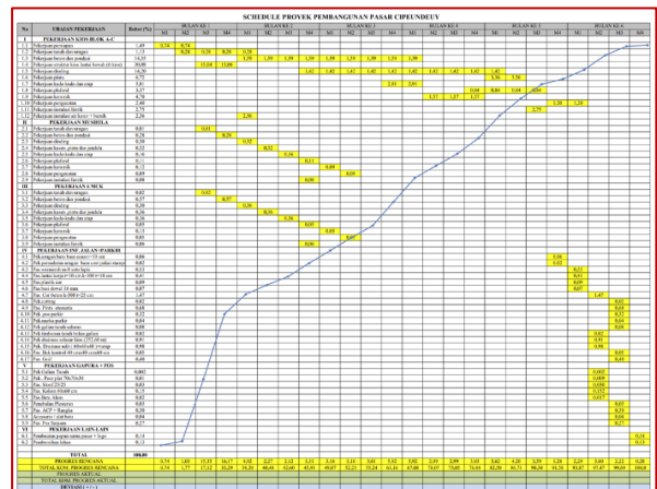
Gambar 4. 4 Penjadwalan Kurva S & Gantt Chart
